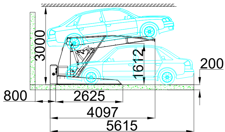
Side View(Sedan-sedan)
