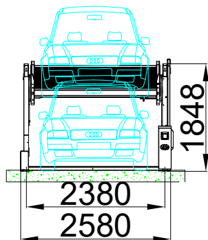
Side View(Sedan-sedan)
